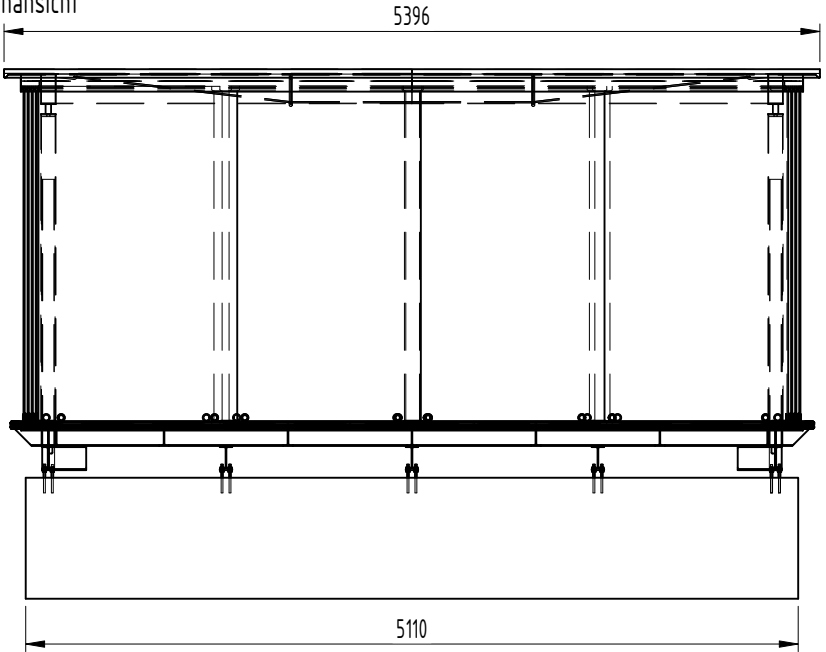
Seitenansicht
