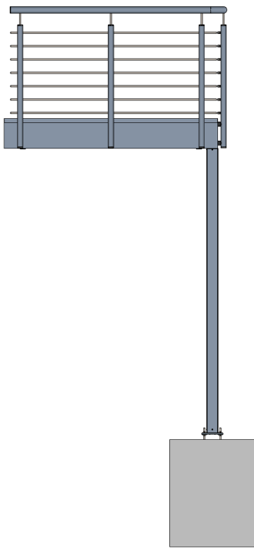
Seitenansicht
