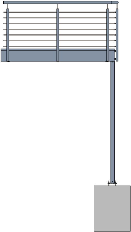
Seitenansicht
