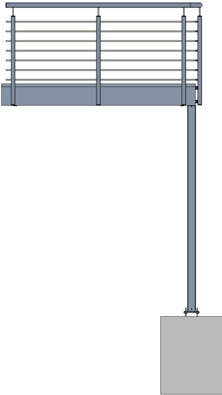
Seitenansicht
