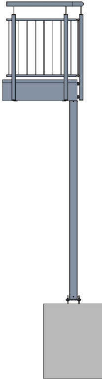
Seitenansicht
