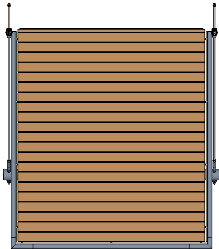
Draufsicht
