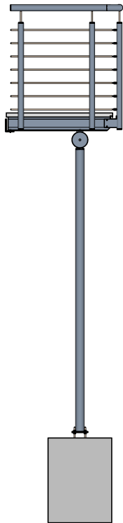
Seitenansicht
